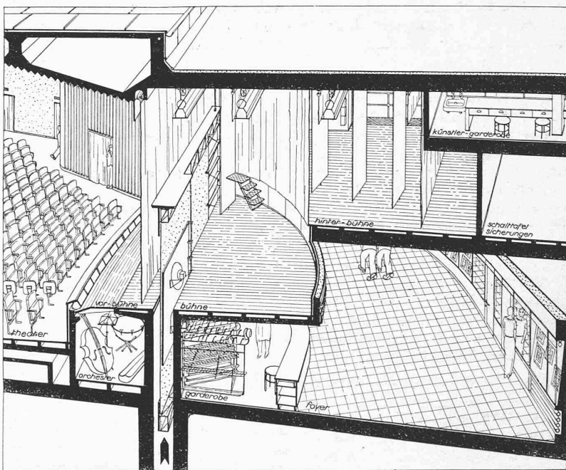
Abb. 11. Perspektivischer Schnitt durch Kino-Bühne und Foyer.
