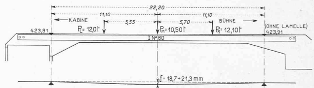
Abb. 45. Durchbiegung der Schiebedach-Laufbahnträger. 1 : 350.
