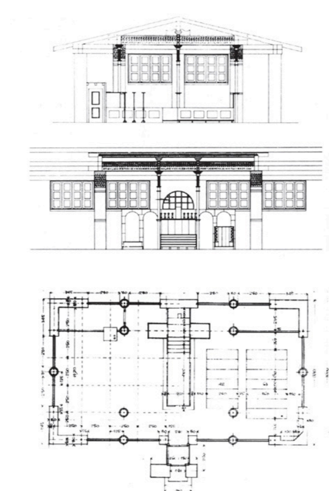
Plan et coupes de l'église
